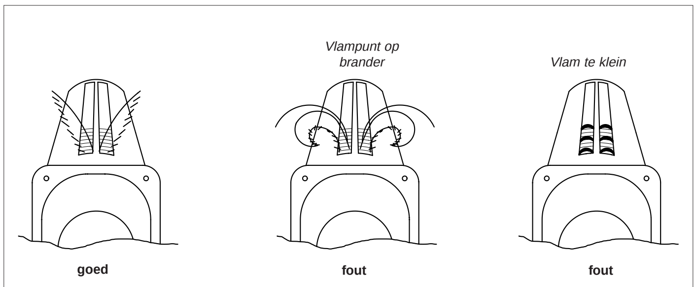
Afb. 13 Controle van het vlambeeld
