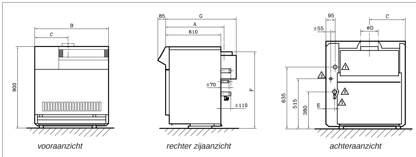
Afb. 02 Afmetingen remeha Gas 1020
