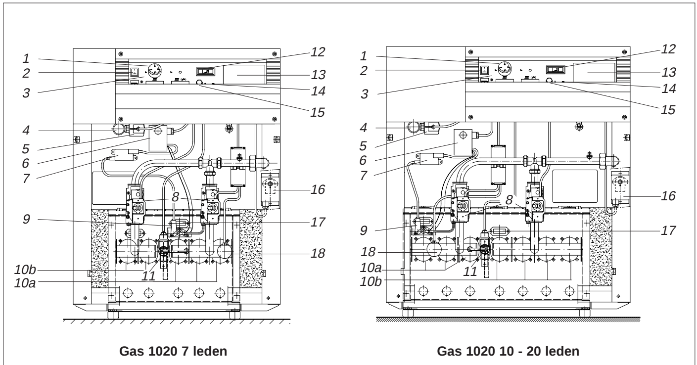
Afb. 04 Regel- en beveiligingsapparatuur
