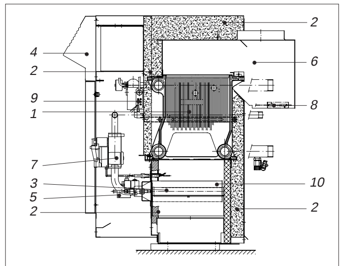
Afb. 01 Doorsnede
