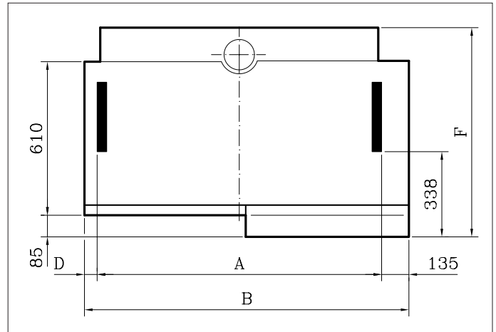
Afb. 06 Steunoppervlak 7 t/m 14 leden
