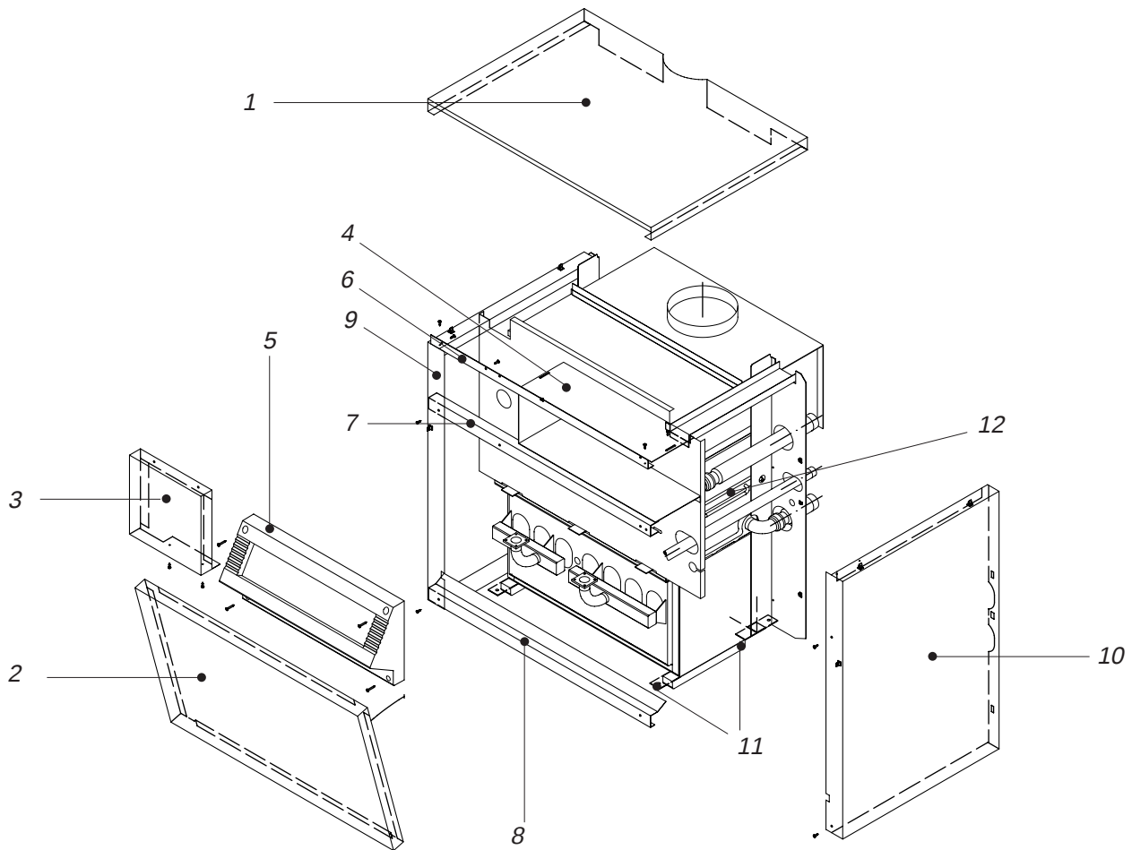
Afb. 08 Demontagevoorschrift
